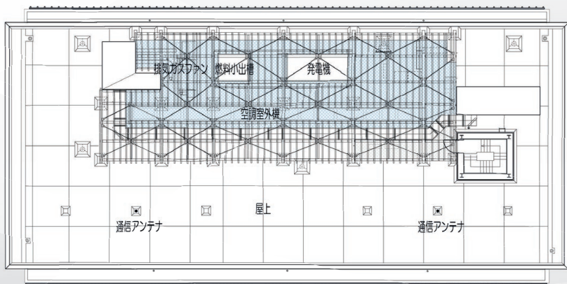
屋上階平面
