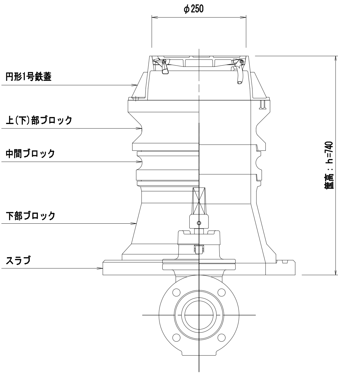
仕切弁BOX積上表（円形1号）
