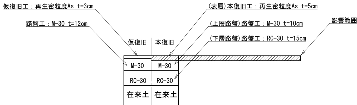
市道 復旧・本復旧
