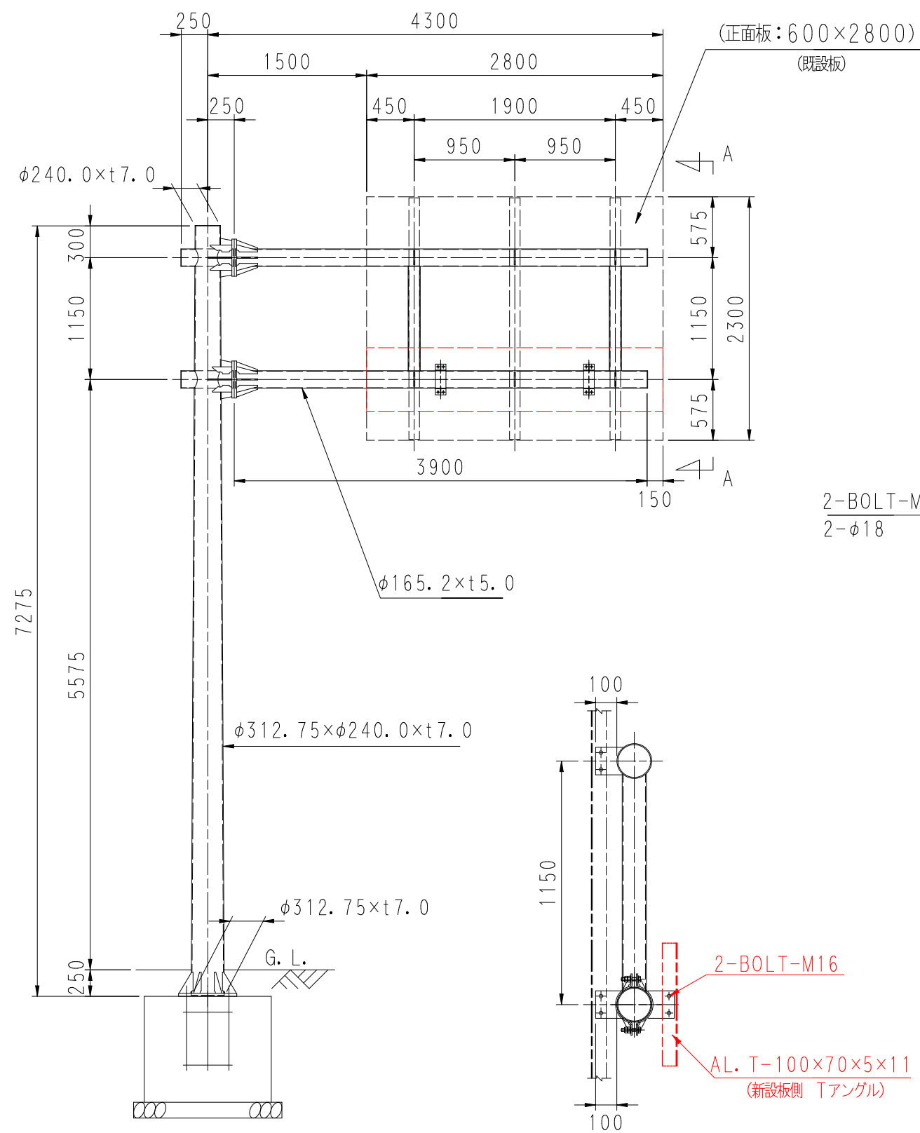
F型構造図 (B-41) S=1/50 (近畿地整)
