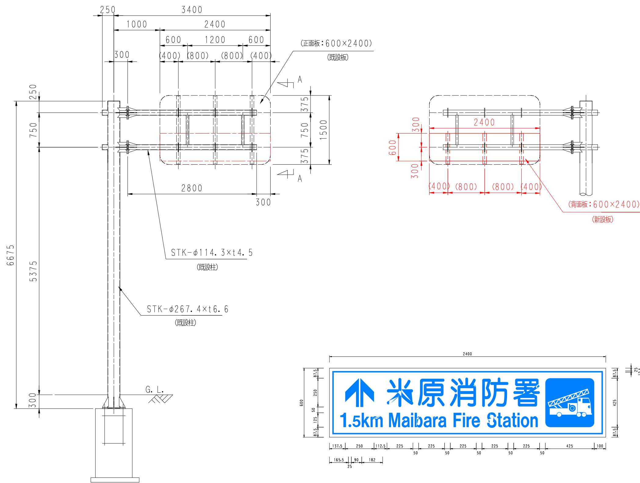
F型構造図 S=1/50
