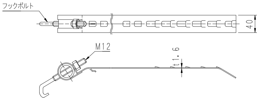
腕金具 SID-18 S=1/5
