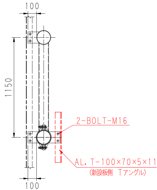
標識側面図 S=1/25 A-A矢視図
