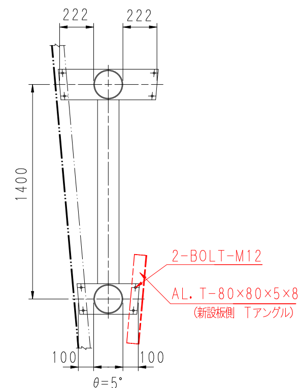
標識側面図 S=1/25
