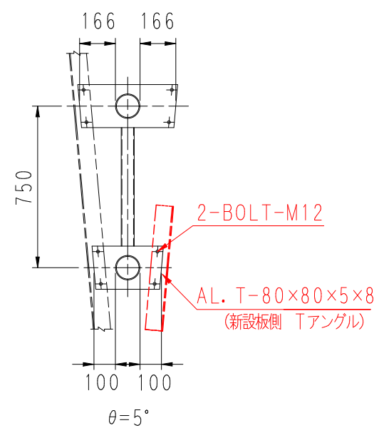
板取付金具詳細図 S=1/25 A-A矢視図
