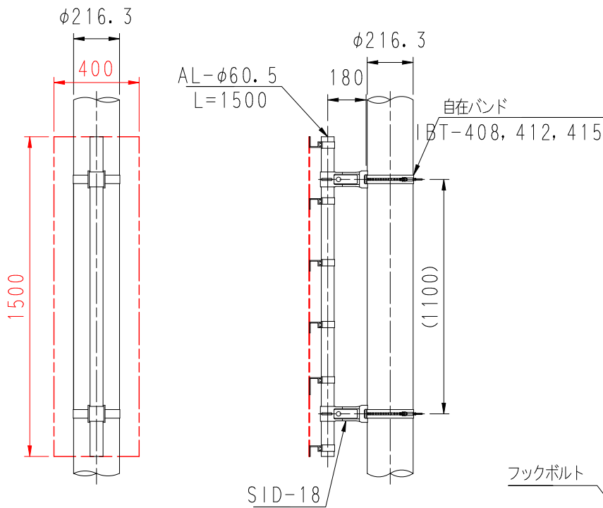
板取付金具詳細図 S=1/25
